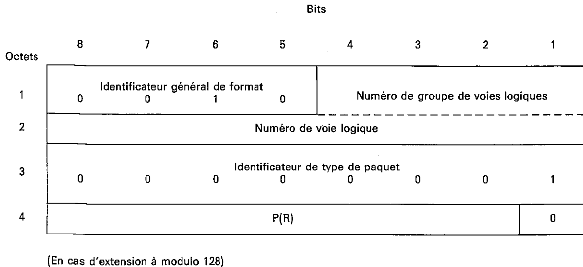
FIGURE 13/X.25 Format des paquets RR de l'ETTD ou l'ETCD
